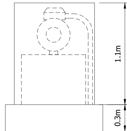
END ELEVATION
